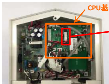
図2. 正面ふたを開いた状態
